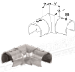
Rohrverbinder 90° horizontal
