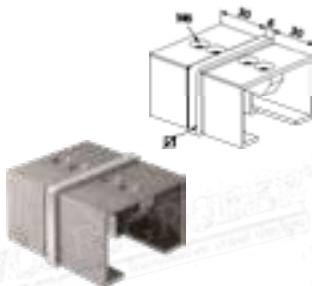
Rohrverbinder
